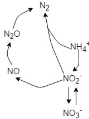
Figura 1. Conversiones biológicas del nitrógeno
