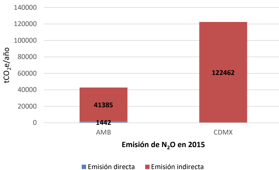
Figura 4. Emisión directa e indirecta del AMB y CDMX en 2015 con la metodología del IPCC
