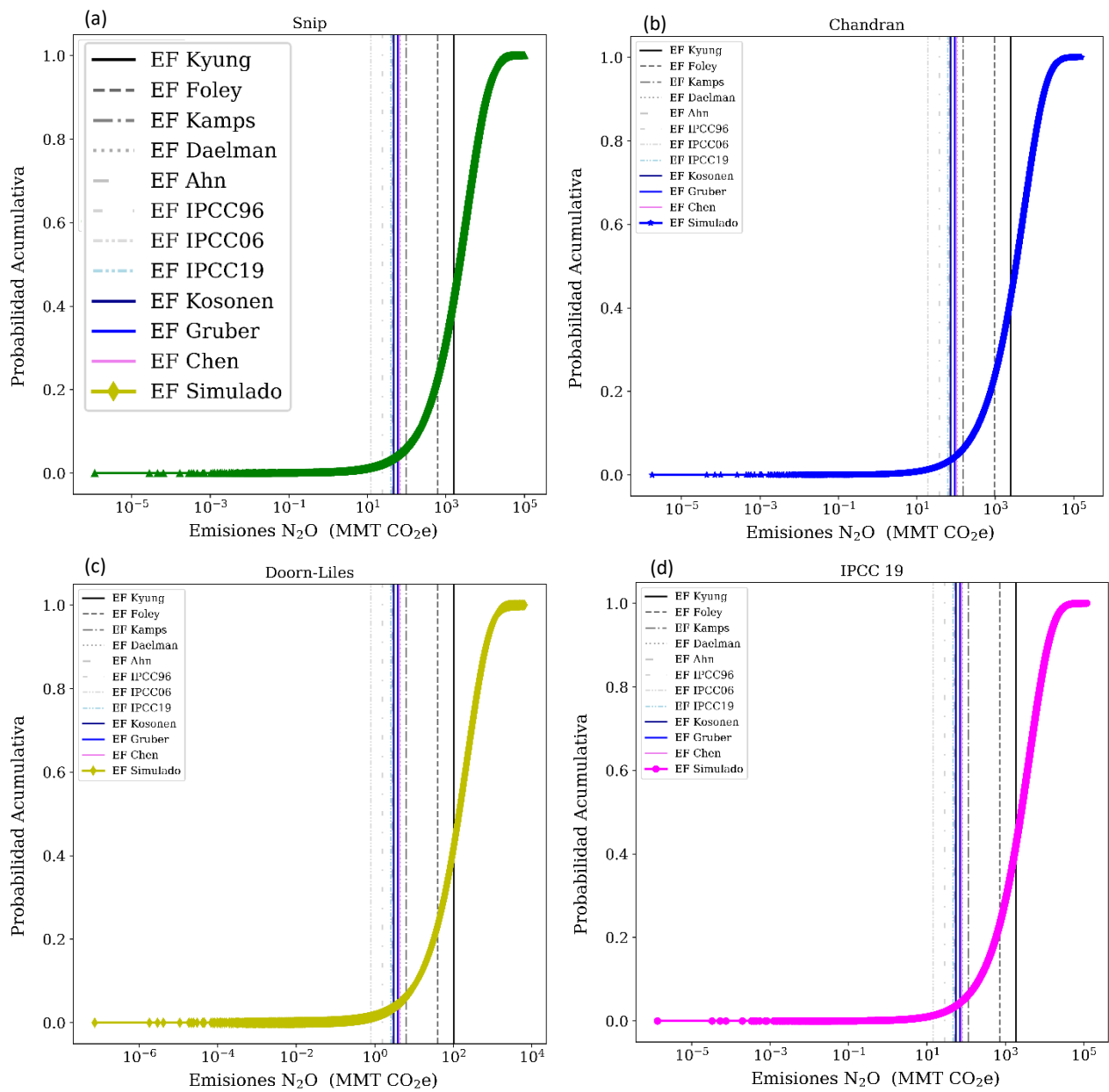
Figura 9. Resultados basados en la probabilidad acumulativa de emisión de N_2O del tratamiento de aguas residuales con las metodologías de IPCC (2019), Snip, Chandran y Doorn-Liles
