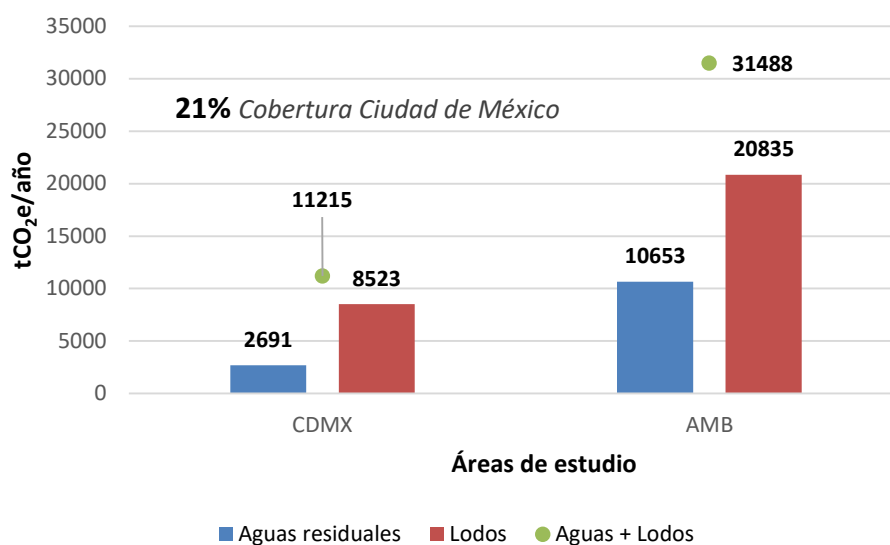
Figura 5. Emisión de CDMX y el AMB en 2015 con las metodologías integradas de Doorn-Liles y Lara-Préndez
