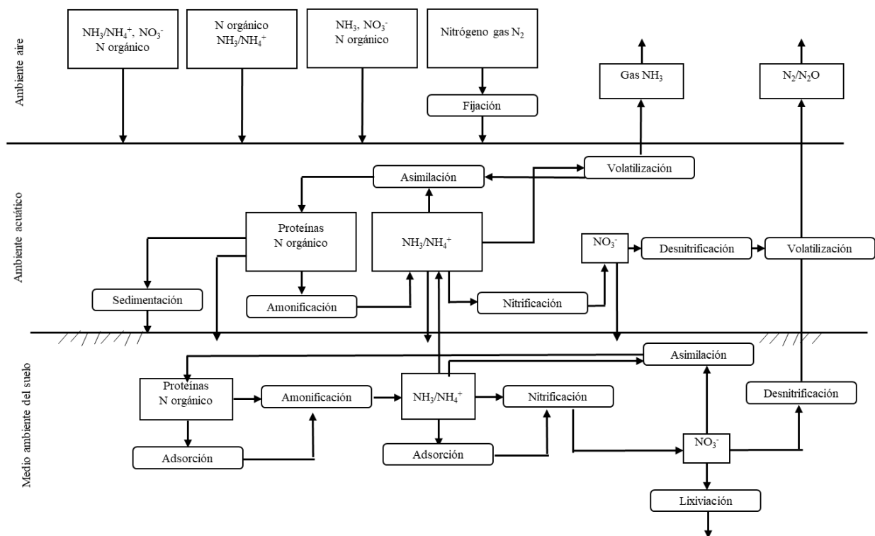
Figura 3. Ciclo del nitrógeno generalizado en el medio ambiente (Metcalf & Eddy et al. , 2014a)
