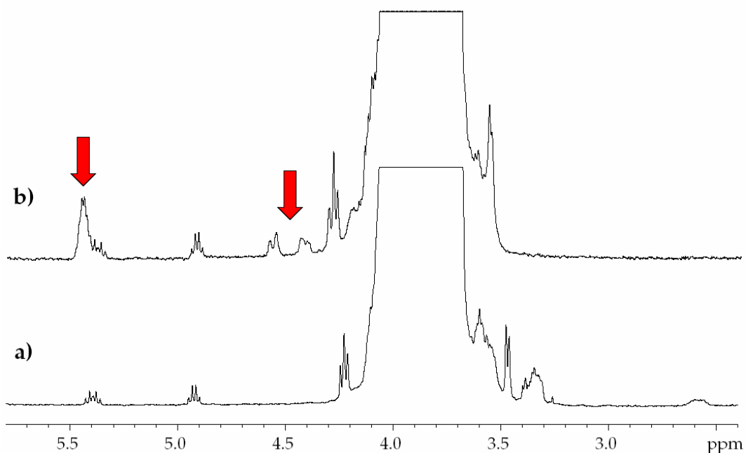
Figura 2.54.- Fragmento del espectro de RMN de ^1\text{H} , registrado en \text{CDCl}_3 , del PFGE obtenido con \text{K } \textit{terc}\text{-BuO} (a) y a los 5 min. de añadir un exceso de TFAA (b).
