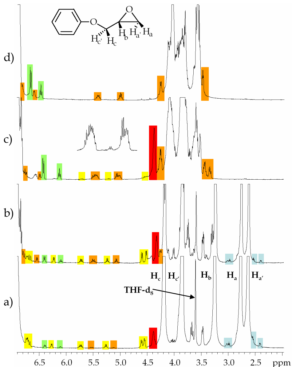
Figura 2.25.- Ampliación del espectro de RMN de 1 H de la mezcla de FGE/K tert -BuO (2:1) en THF-d 8 calentada a 60°C. a) Después de 20 min., b) a los 40 min., c) a los 60 min. y d) después de la adición de H 2 SO 4 en D 2 O.
