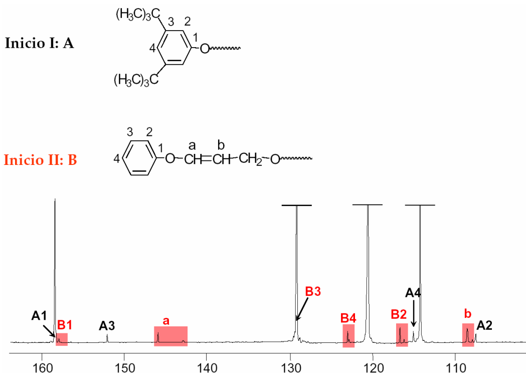
Figura 2.42.- Ampliación de la región aromática del espectro de RMN de ^{13}\text{C} del PFGE obtenido con el sistema iniciador 3,5-di- tert -butilfenol/ t -Bu- \text{P}_4 (1:1).
