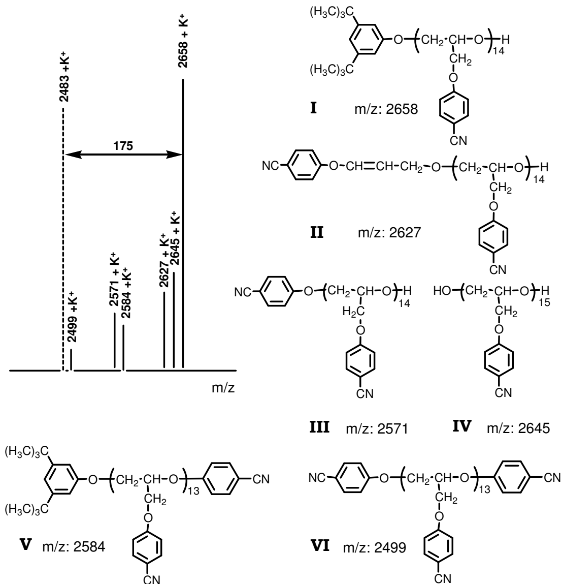
Figura 2.34.- Representación del patrón repetitivo observado en los picos del MALDI-TOF MS del poli(4-CN-FGE) obtenido con el sistema 3,5-di- terc -BuPhOH/ t -bu P 4 .
