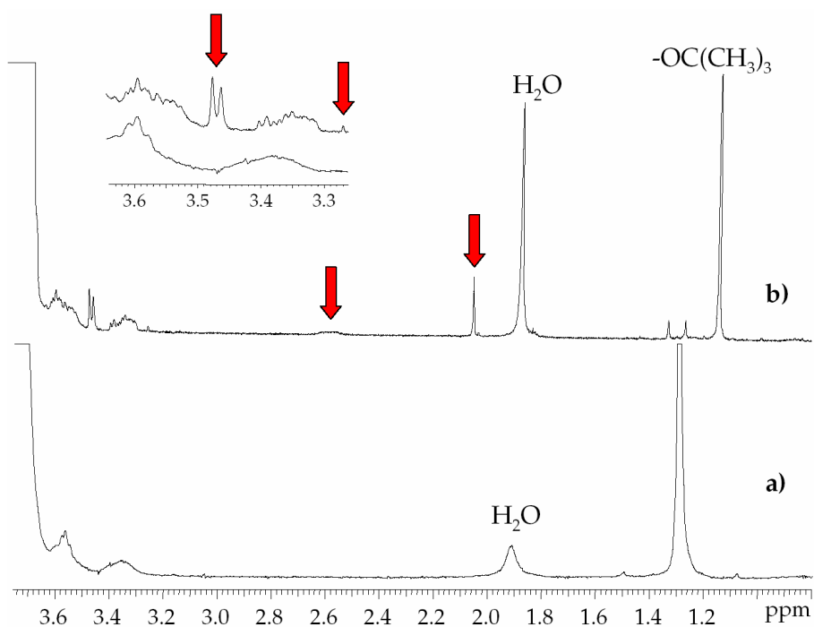
Figura 2.53.- Fragmento de los espectros de RMN de 1 H pertenecientes al PFGE obtenido con sistema iniciador 3,5-di- tert -butilfenol/t-Bu-P 4 ( a ) y del PFGE obtenido utilizando el K tert -BuO ( b ).
