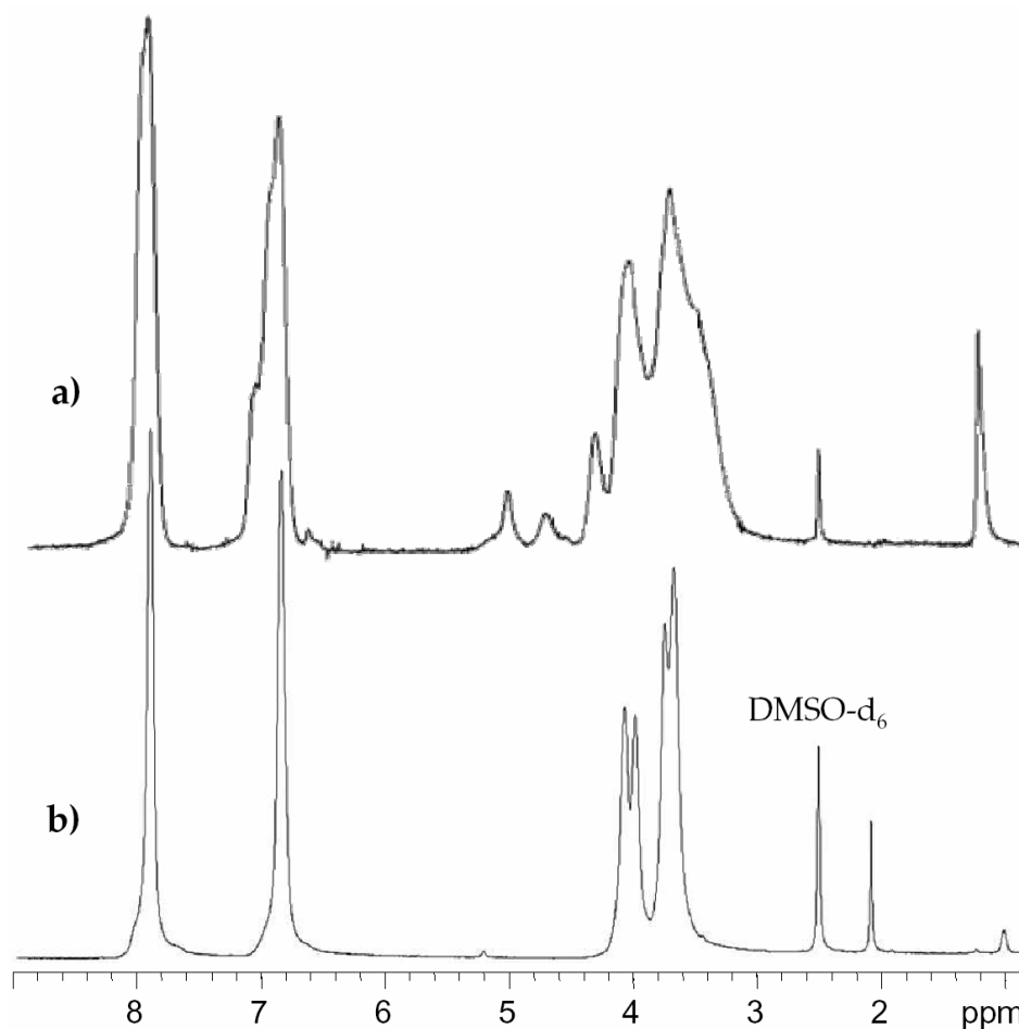
Figura 2.50.- Espectros de RMN de ^1\text{H} de los Poli(4- \text{NO}_2 FGE) obtenidos con el sistema iniciador 3,5-di- terc -butilfenol/ t -Bu \text{P}_4 (1:1) (a) y con el catalizador de Teyssié (b).
