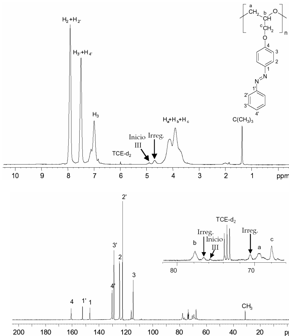
Figura 2.36.- Espectros de RMN de 1 H y 13 C registrados en TCE-d 2 , del poli(4-C 6 H 5 -N=N-FGE) obtenido con el sistema iniciador 3,5-di- terc -BuPhOH/t-Bu-P 4 .
