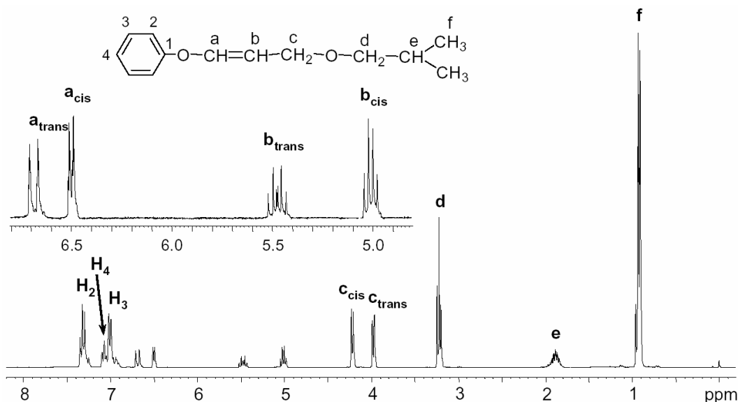
Figura 2.39.- Espectro de RMN de 1 H del 1-fenoxi-3-isobutoxiopropeno registrado en CDCl 3 .
