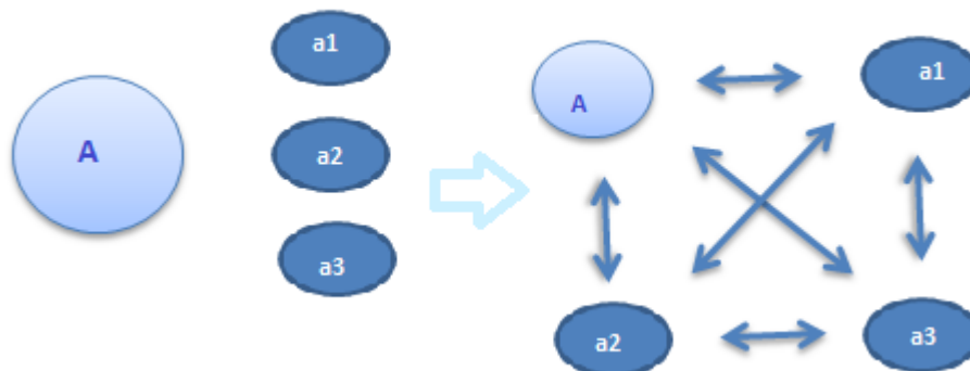
Ilustración 3: Aprendizaje combinatorio.
