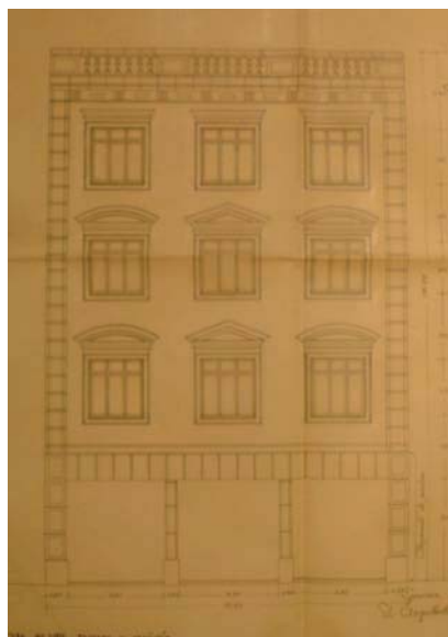
53-Edifici Coll – Maó (1946) Foto plànol del fons Claret (reg. COAC 10035)
