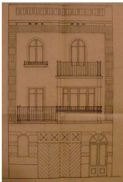
52-Casa Roure – Girona (1948) Foto plànol del fons Claret (reg. COAC 10064)
