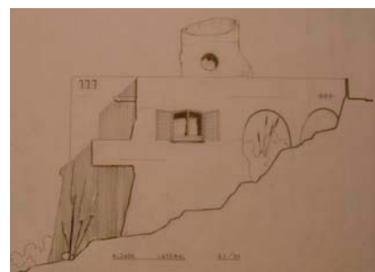
116-Xalet; parc. 241 - Montgó – L’Escala (1974) Fotos plànols del fons Claret (reg. COAC 10220)
