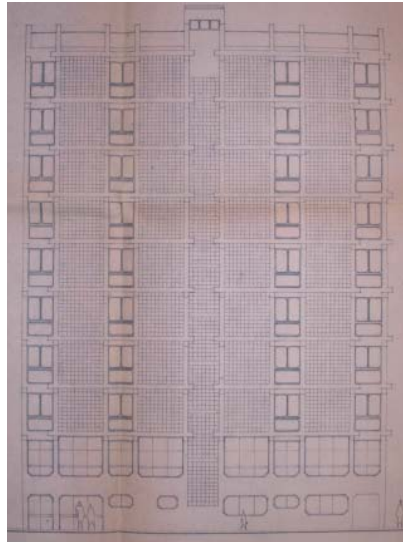
110-Habitatges Caixa Pensions - Girona (1966) Foto plànol del fons Claret (reg. COAC 10198)
