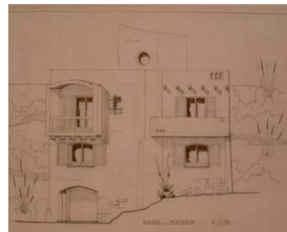
115-Xalet Gisa; parc. 5 - Montgó – L’Escala (1974) Fotos plànols del fons Claret (reg. COAC 10232)
