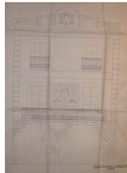
79-Edifici Ajuntament – Amer (1956) Foto plànol del fons Claret (reg. COAC 10024)
