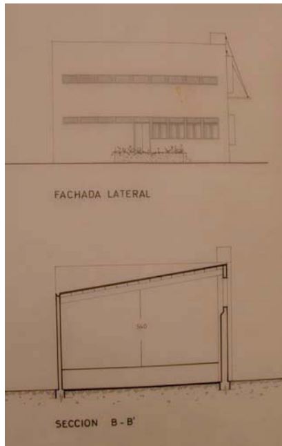
132-Magatzem Esteban – Palafolls (sd) Fotos plànols del fons Claret (reg. COAC 2147)
