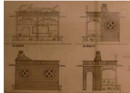
44-Botiga Pujadas – Girona (1947) Foto plànol del fons Claret (reg. COAC 10067)
