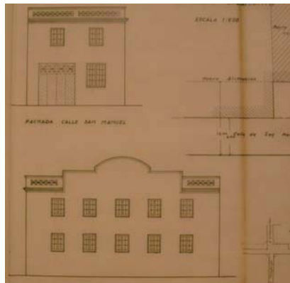
59-Casa Cornellà – Girona (1946) Foto plànol del fons Claret (reg. COAC 10115) i foto de l'estat actual
