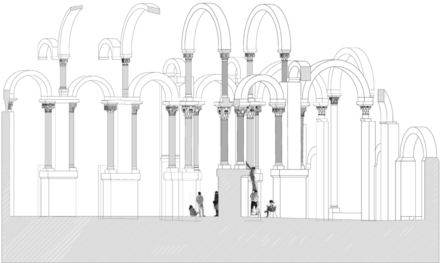
Il·lustració 292: església de Sant Pere de Rodes, secció obliqua.
