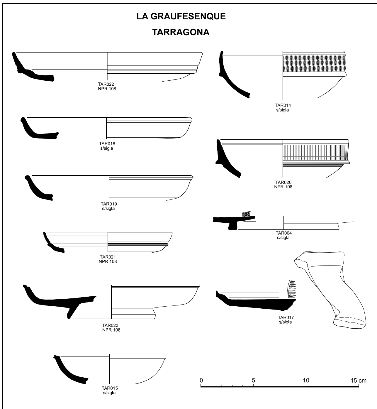
Figura 175. Individus de Tarraco analitzats, associats a la producció de terra sigillata de La Graufesenque
