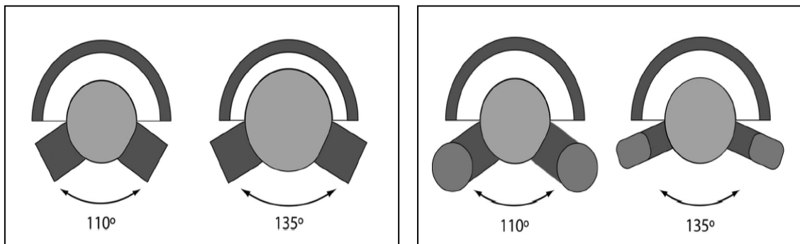
Fig.36 Aumento del rango de movimiento por el aumento del tamaño de la cabeza femoral (izquierda) y por el cambio de geometría del cuello (derecha) de circular a trapecoidal. 101
