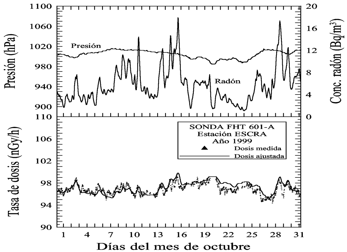
Figura B.10: Comparación entre la tasa de dosis medida en la estación ESCRA y la tasa de dosis ajustada durante el mes de octubre del año 1999. Sonda FHZ601A.
