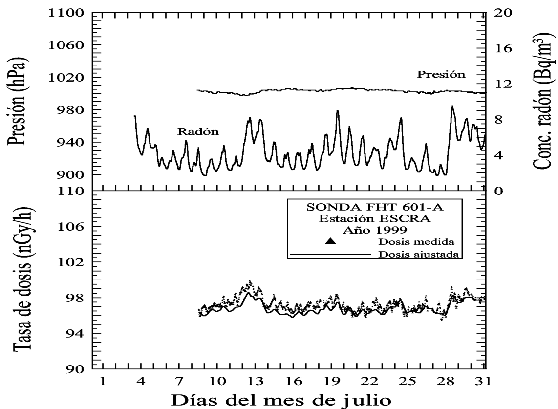
Figura B.7: Comparación entre la tasa de dosis medida en la estación ESCRA y la tasa de dosis ajustada durante el mes de julio del año 1999. Sonda FHZ601A.
