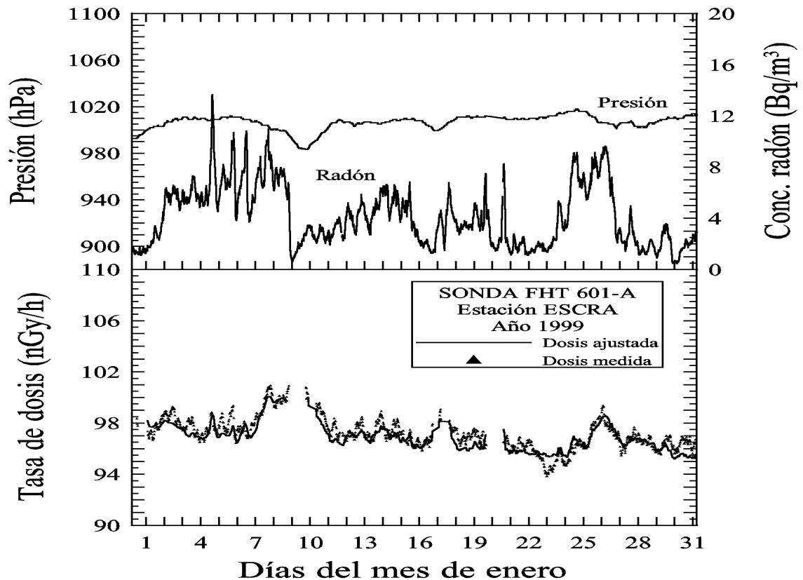
Figura B.1: Comparación entre la tasa de dosis medida en la estación ESCRA y la tasa de dosis ajustada durante el mes de enero del año 1999. Sonda FHZ601A.
