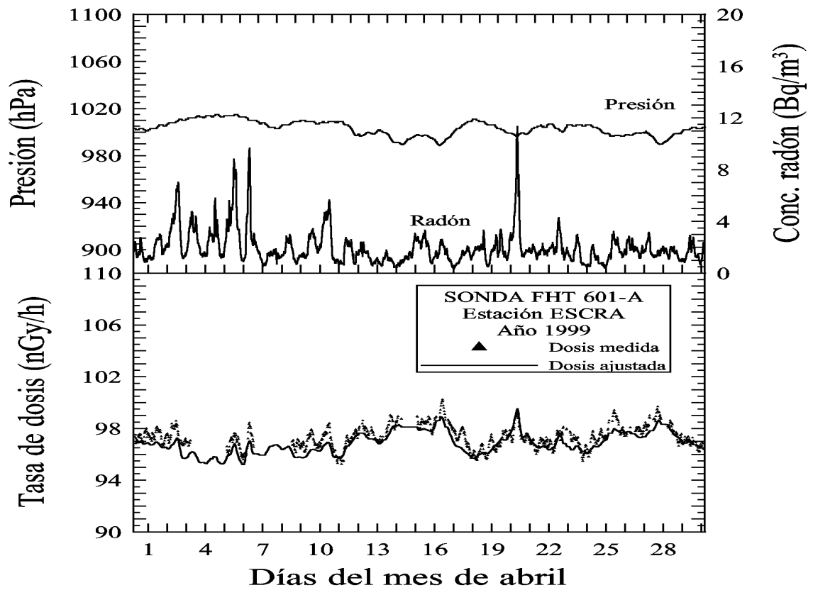
Figura B.4: Comparación entre la tasa de dosis medida en la estación ESCRA y la tasa de dosis ajustada durante el mes de abril del año 1999. Sonda FHZ601A.
