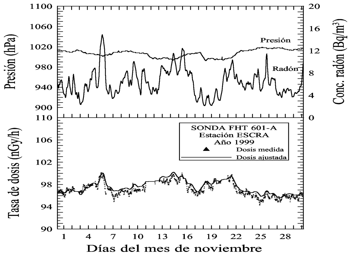
Figura B.11: Comparación entre la tasa de dosis medida en la estación ESCRA y la tasa de dosis ajustada durante el mes de noviembre del año 1999. Sonda FHZ601A.
