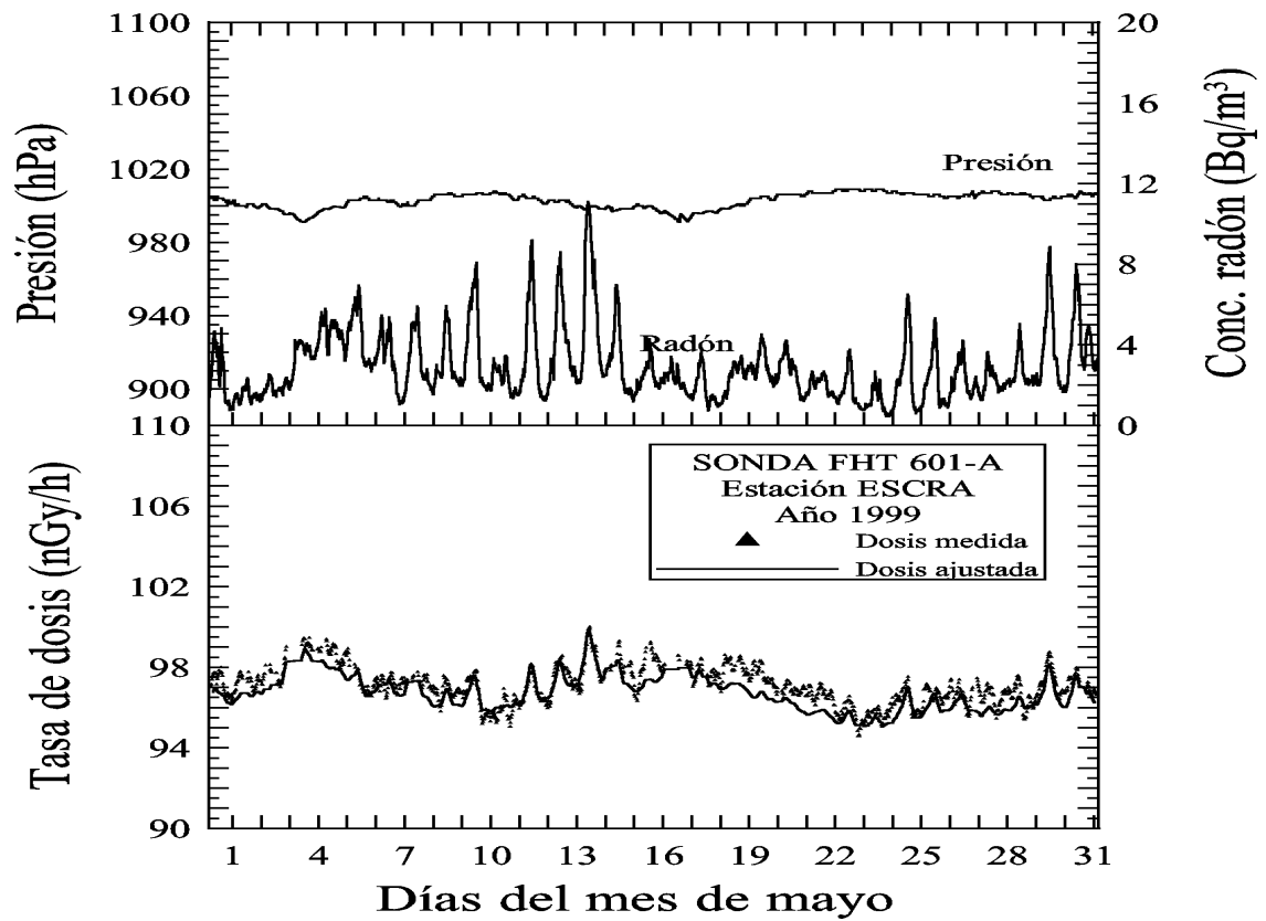
Figura B.5: Comparación entre la tasa de dosis medida en la estación ESCRA y la tasa de dosis ajustada durante el mes de mayo del año 1999. Sonda FHZ601A.
