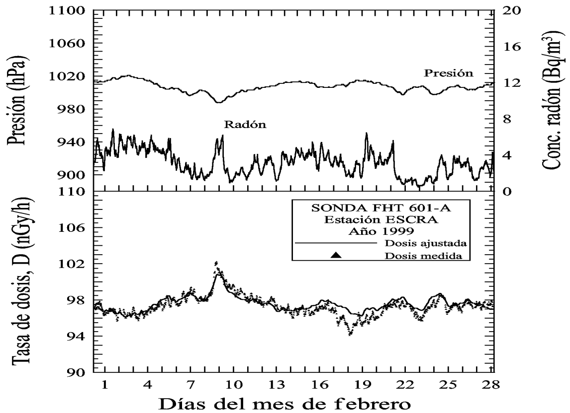
Figura B.2: Comparación entre la tasa de dosis medida en la estación ESCRA y la tasa de dosis ajustada durante el mes de febrero del año 1999. Sonda FHZ601A.
