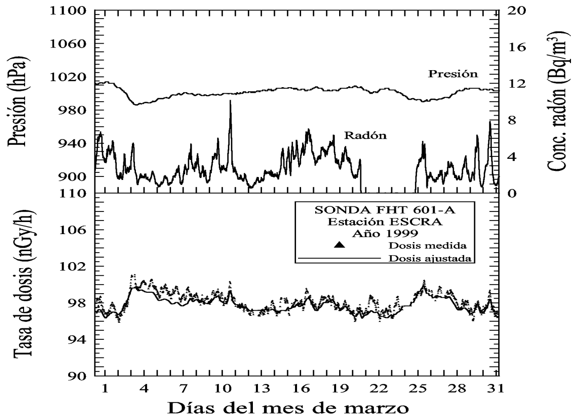
Figura B.3: Comparación entre la tasa de dosis medida en la estación ESCRA y la tasa de dosis ajustada durante el mes de marzo del año 1999. Sonda FHZ601A.
