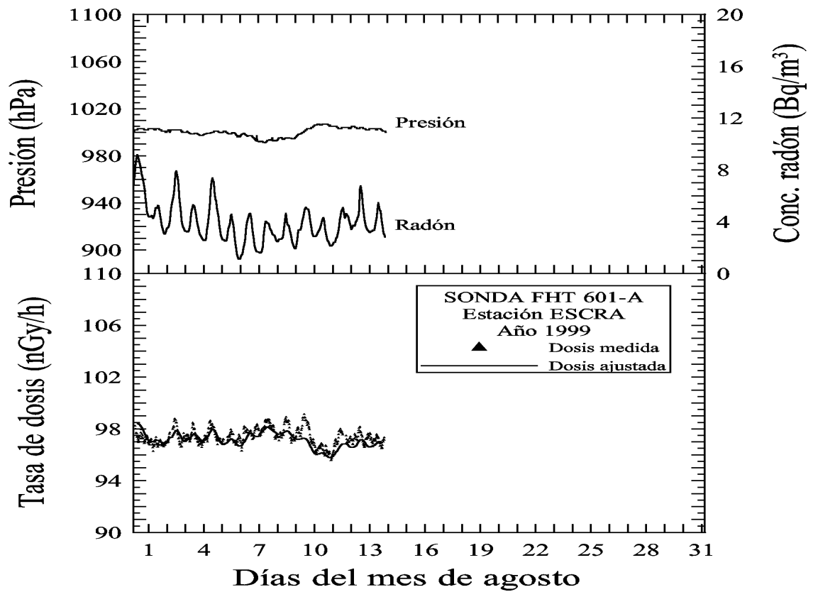
Figura B.8: Comparación entre la tasa de dosis medida en la estación ESCRA y la tasa de dosis ajustada durante el mes de agosto del año 1999. Sonda FHZ601A.
