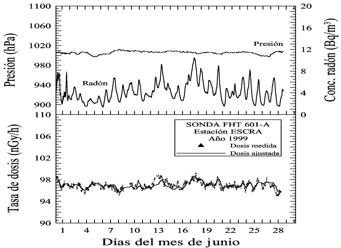
Figura B.6: Comparación entre la tasa de dosis medida en la estación ESCRA y la tasa de dosis ajustada durante el mes de junio del año 1999. Sonda FHZ601A.
