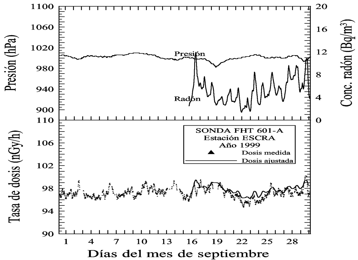
Figura B.9: Comparación entre la tasa de dosis medida en la estación ESCRA y la tasa de dosis ajustada durante el mes de septiembre del año 1999. Sonda FHZ601A.
