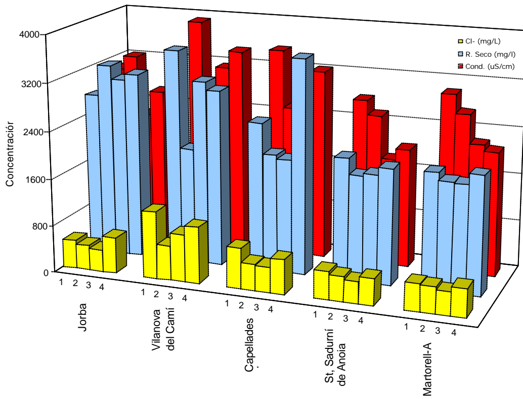
Figura 15: Evolución espacial y temporal de cloruros, residuo seco y conductividad en el río Anoia
