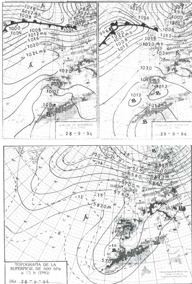
Figura 6.66.- Análisis en superficie y en altura del episodio 28-29.09.94 (INM, 1994).
